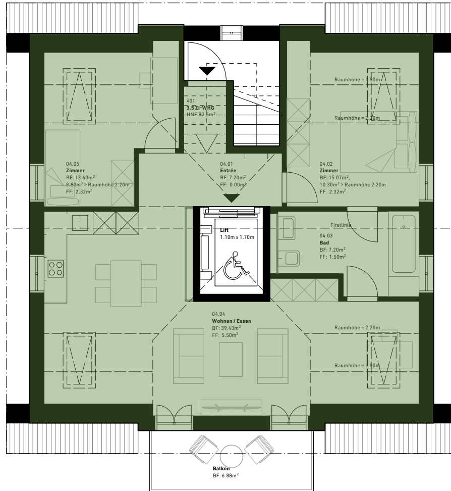
Dachgeschoss Mst. 1:100
