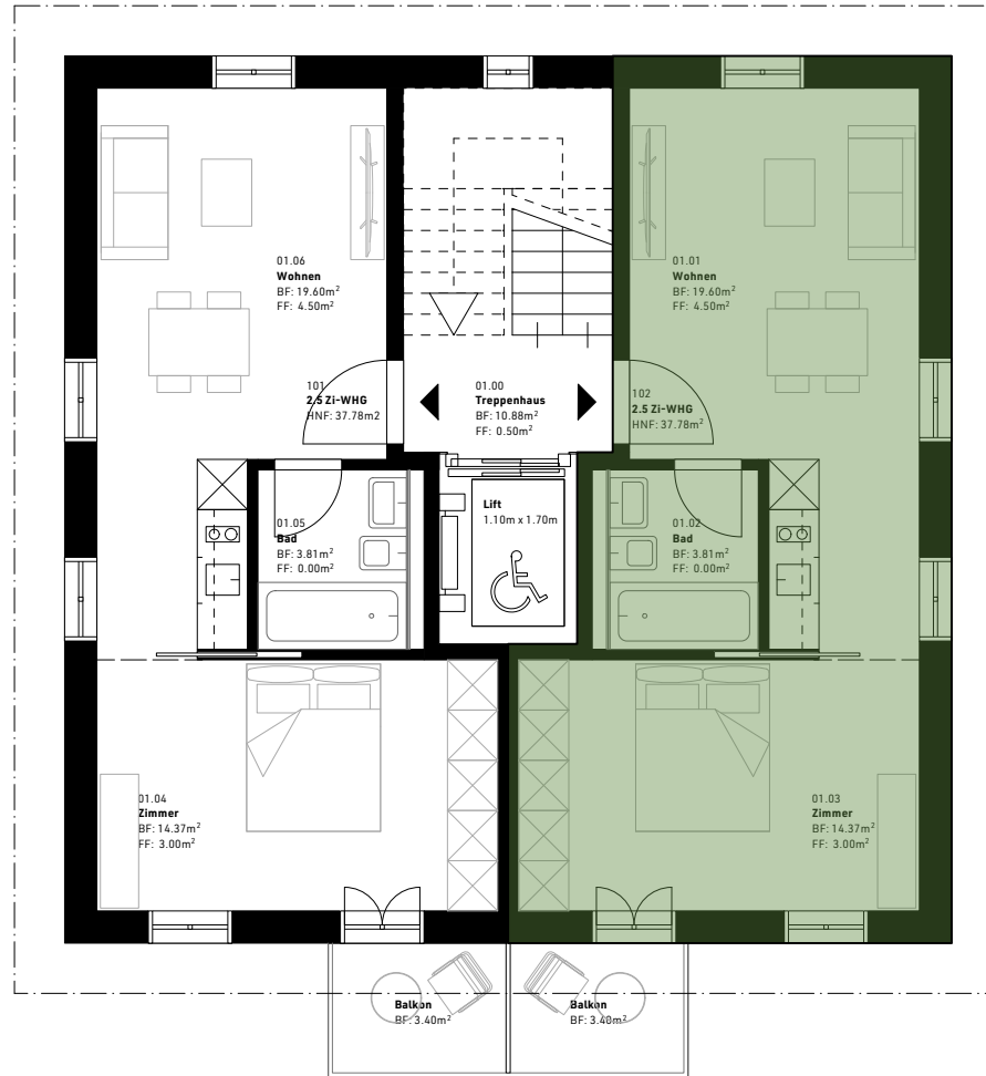
2.Obergeschoss Mst. 1:100
