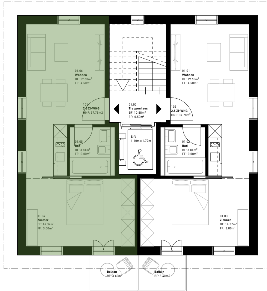
3.Obergeschoss Mst. 1:100
