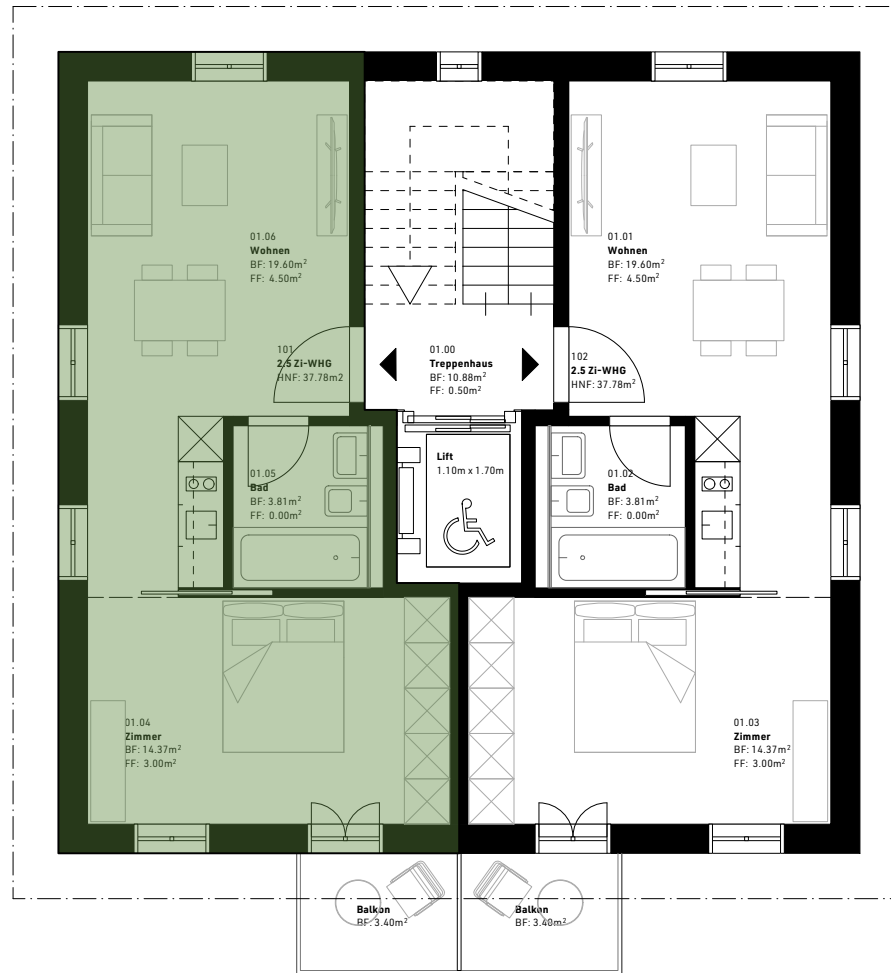
1.Obergeschoss Mst. 1:100
